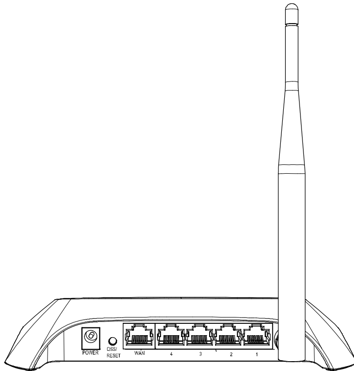
图 3-2 TL-WR740N 后面板示意图
