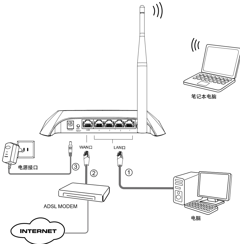
图 4-1 TL-WR740N 硬件安装示意图
